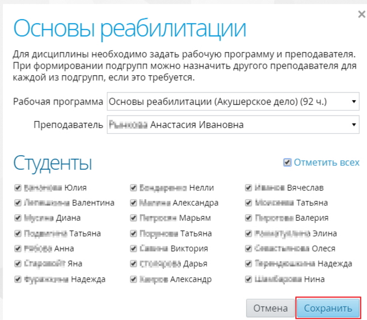
Рисунок 180. Сохранение параметров
