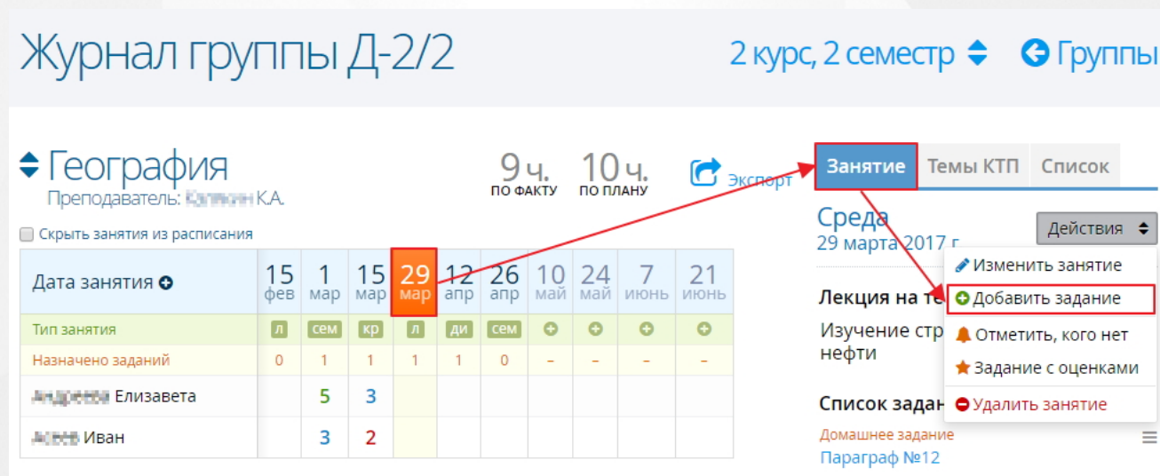
Рисунок 238. Добавление задания
