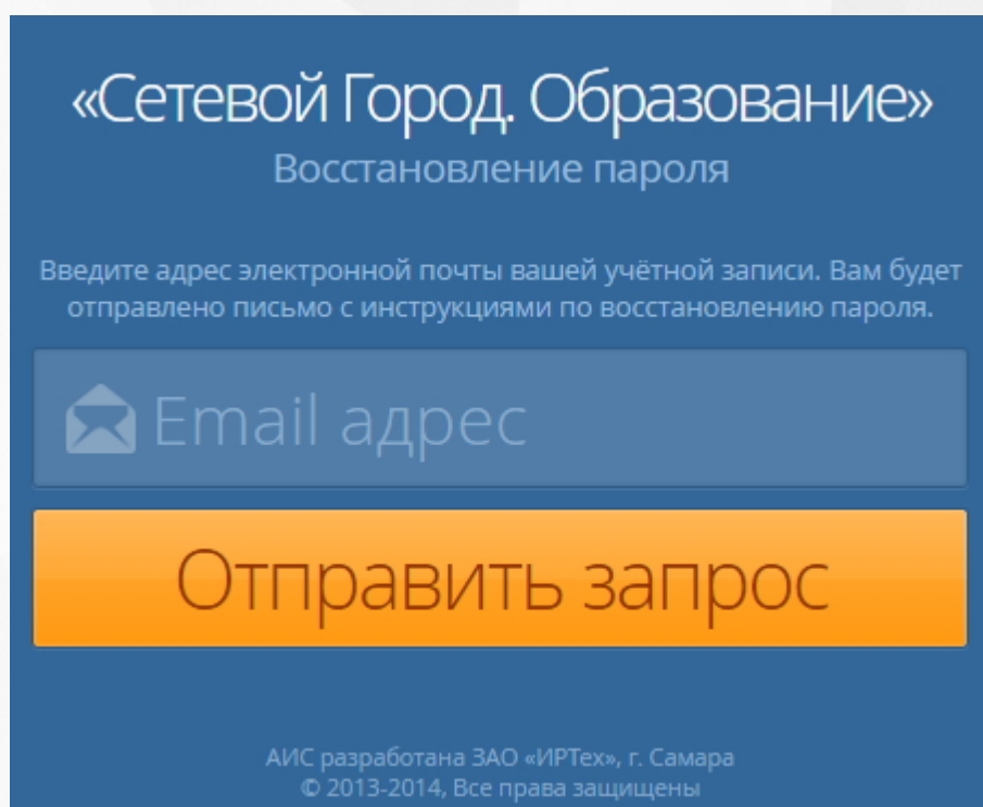
Рисунок 52. Восстановление пароля
