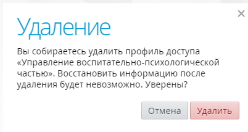
Рисунок 33. Удаление профиля
