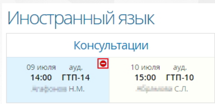
Рисунок 224. Удаление консультации
