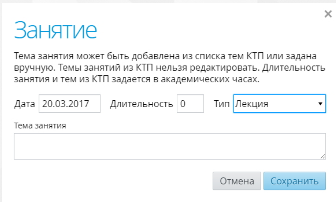
Рисунок 234. Окно «Занятие»
